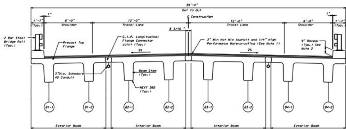
Figure 5 SCALE: 1/2" = 1'-0"
