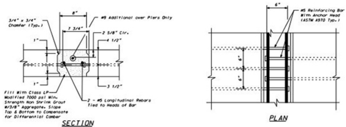
Figure 6 SCALE: 2" = 1'-0"
